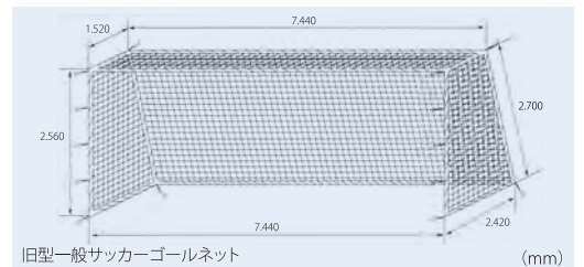
旧型一般サッカーゴールネット (mm)
