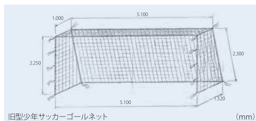
旧型少年サッカーゴールネット
