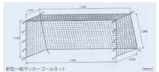
新型一般サッカーゴールネット (mm)
