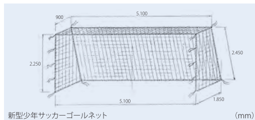
新型少年サッカーゴールネット
